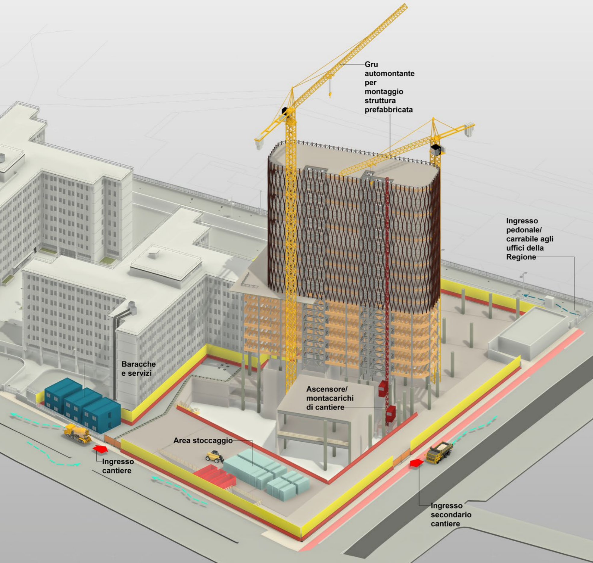
SCHEMA ORGANIZZAZIONE DEL CANTIERE
