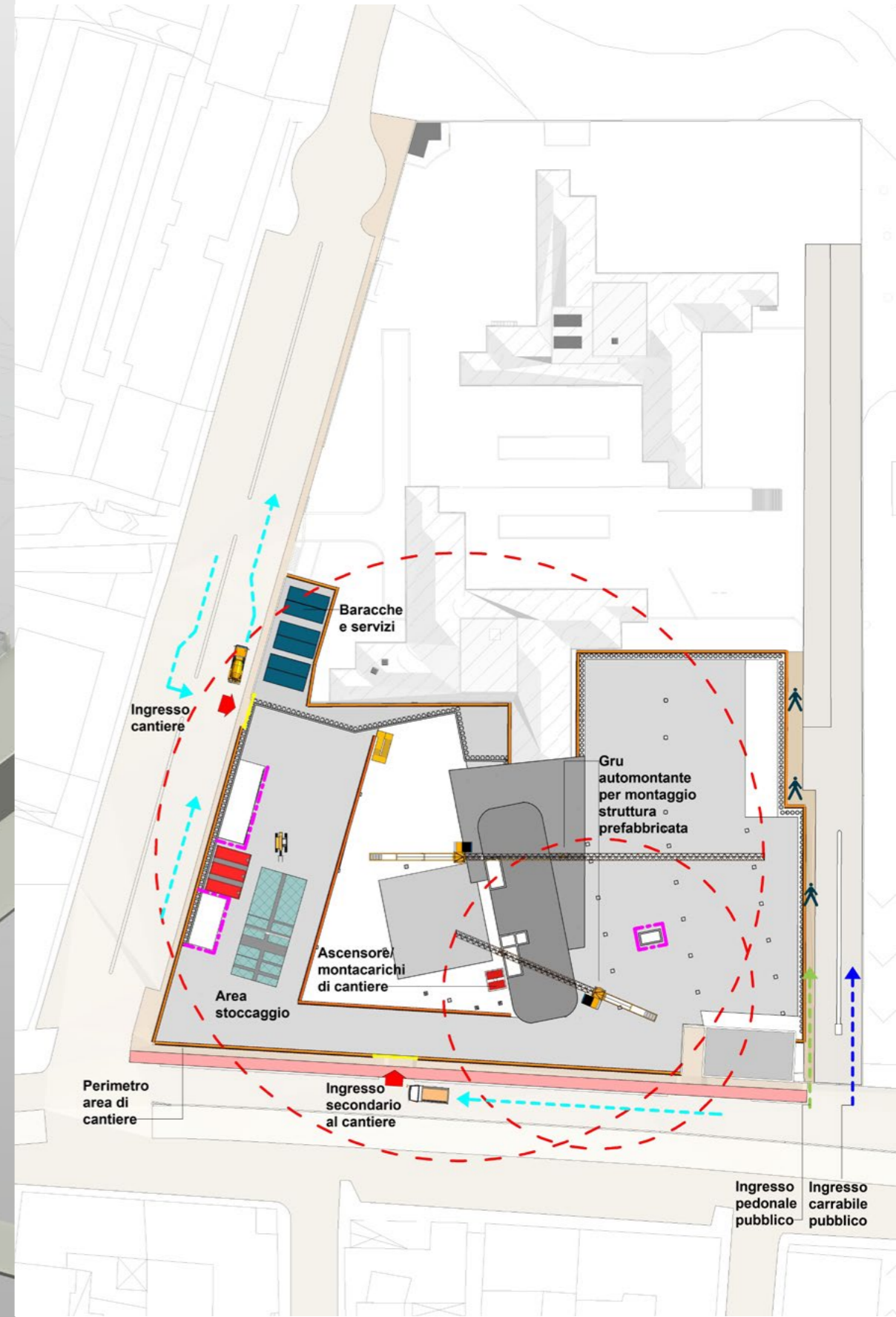
PIANTA CON ORGANIZZAZIONE DEL CANTIERE
